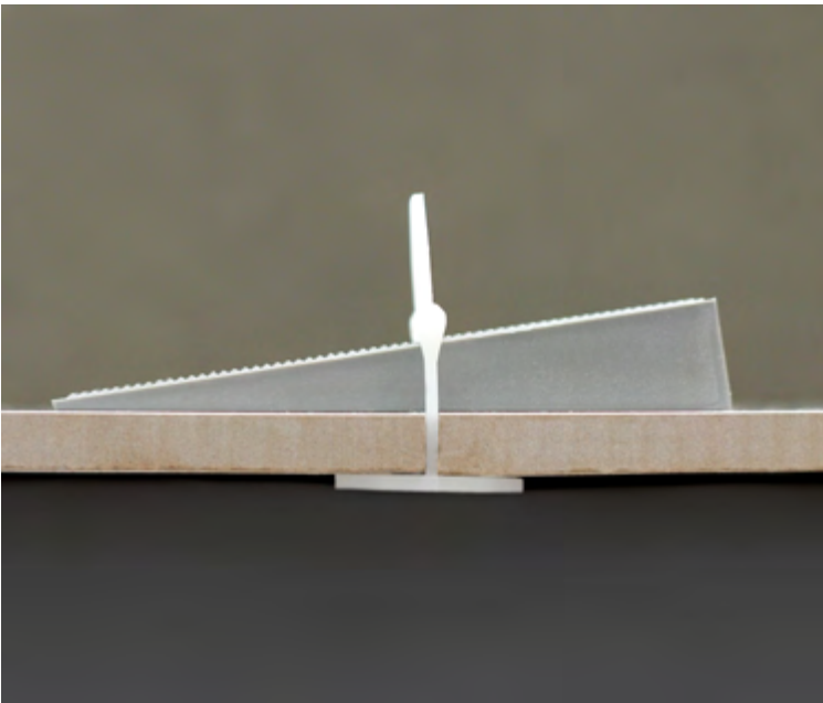
Clipe Nivelador e Cunha já alinhados com o auxílio do Alicate. Leveling Clip and Wedge already aligned with the help of the Pliers. Clipe Nivelador y Cuña ya alineados con la ayuda del Alicate.
